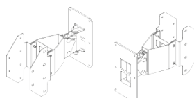
Schwenk-/Neigehalter für zwei Lautsprecher
