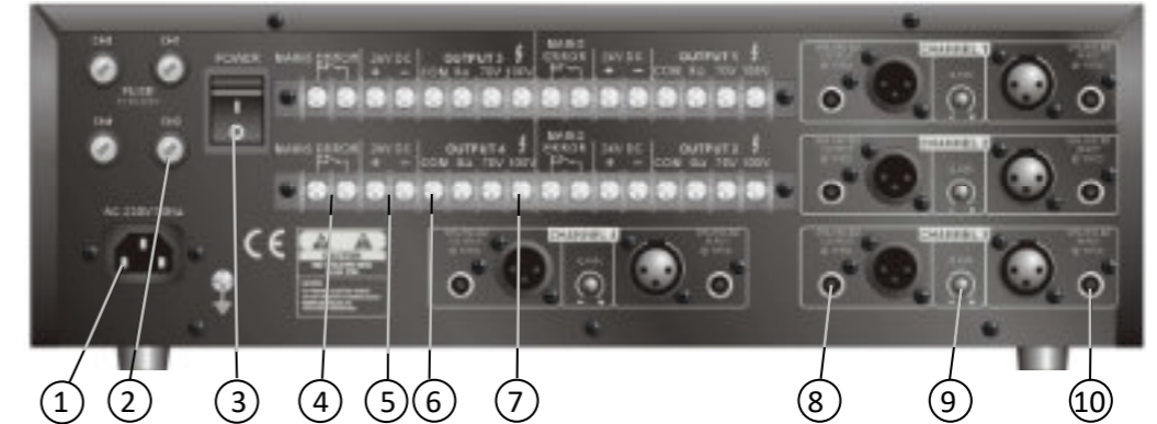
SINUS 220 amplifier:
